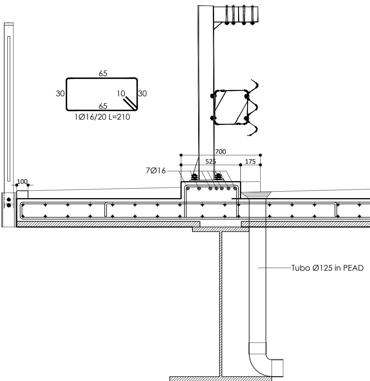
SEZIONE B-B (Scala 1:20)
