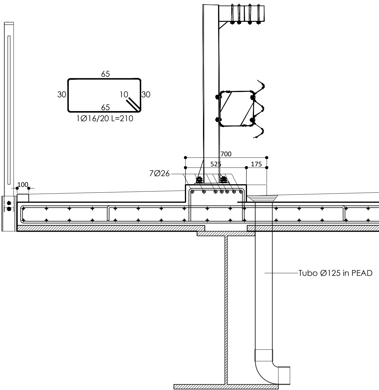
SEZIONE A-A (Scala 1:20)
