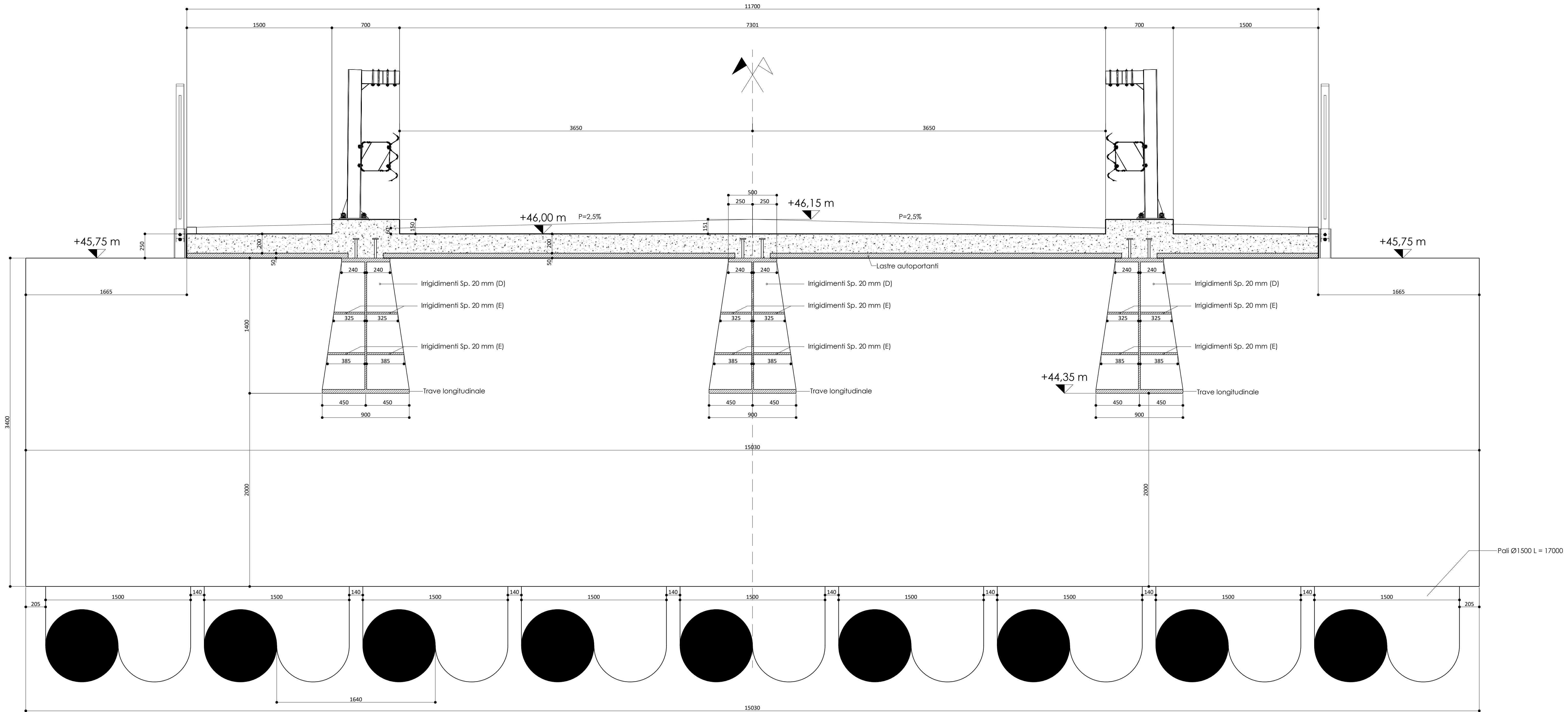
SEZIONE D-D SULLA SPALLA (Scala 1:20)
